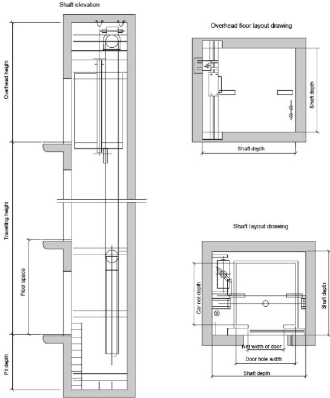
Machine room-less elevator parameter table
